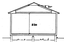
SEKTION
