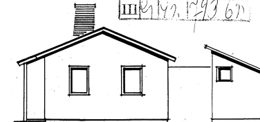
FASAD MOT VÄSTER
